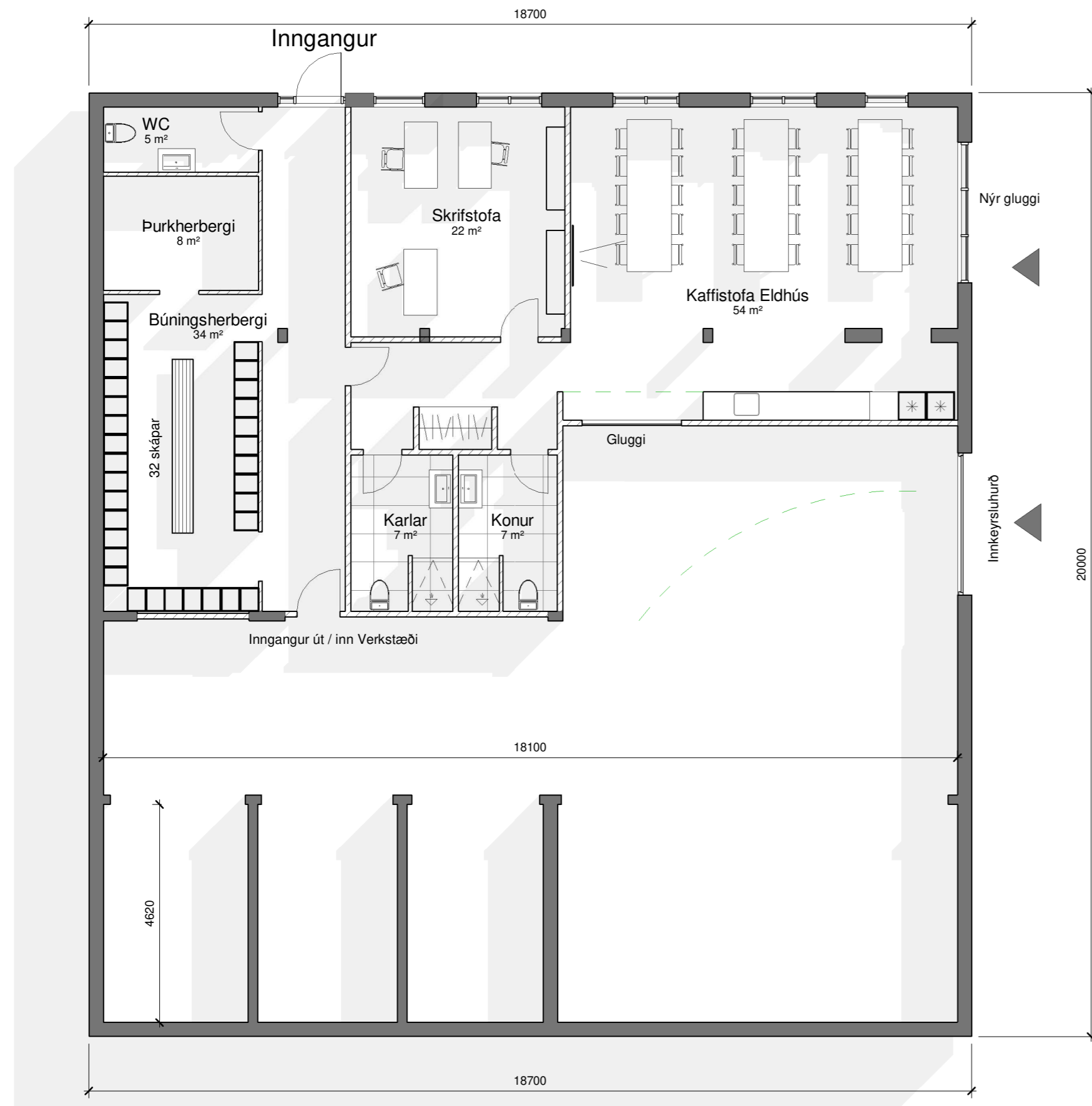
E01 Grunnmynd Mál : 1 : 100
