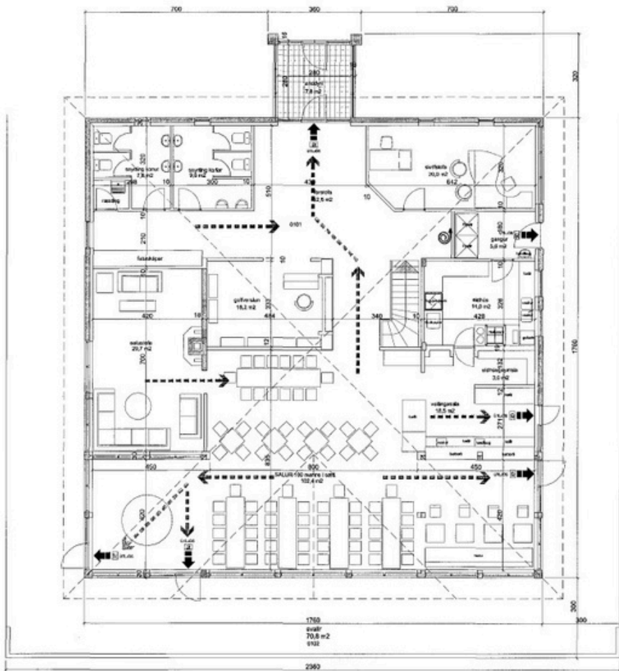
GRUNNMYND 1. HÆÐAR 1:100
